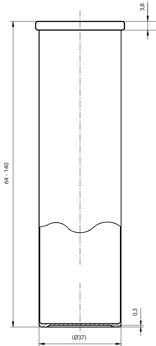
zylindrische Dose mit Sonderformrand
