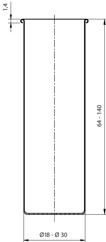
zylindrische Dose mit Außenrollrand
